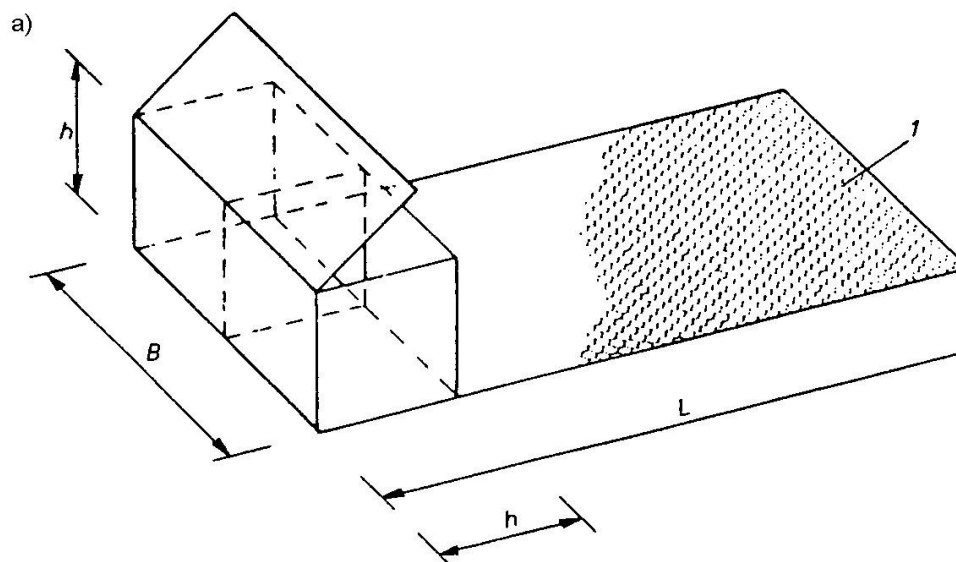
Rys. 12. Konstrukcja siatkowa gabionu, stosowana do wykonania nasypu z gruntu zbrojonego a) Kosz gabionu z siatką zbrojącą grunt, b) Schemat budowli z gruntu zbrojonego o pionowej ścianie czołowej, c) Schemat budowli z gruntu zbrojonego o pochylonej schodkowo ścianie czołowej 1 – Element przedłużający dno kosza (siatka zbrojąca nasyp), 2 – Geowłóknina uszczelniająca kosz gabionu przed zanieczyszczeniem gruntem, 3 – Nasyp ziemny
