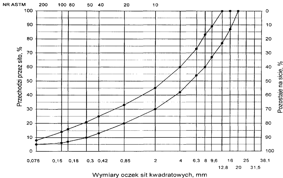
Rys. 13. Krzywe graniczne uziarnienia mieszanki mineralno-asfaltowej BA od 0 do 16 mm do warstwy wyrównawczej nawierzchni drogi o obciążeniu ruchem od KR3 do KR6
