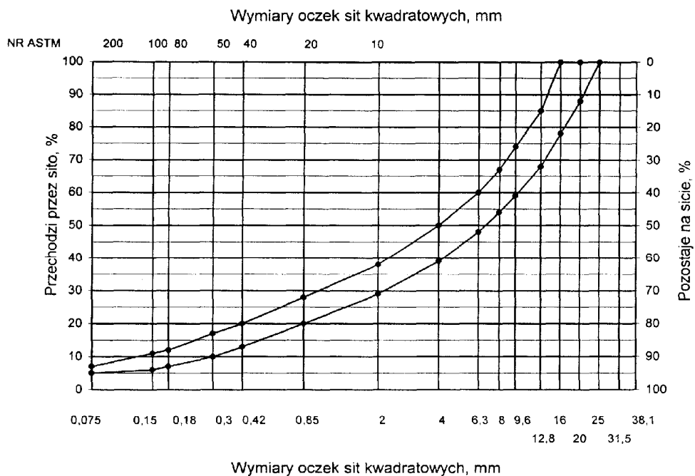
Rys. 3. Krzywe graniczne uziarnienia mieszanki mineralnej BA od 0 do 8mm, od 0 do 6,3 mm do warstwy ścieralnej nawierzchni drogi o obciążeniu ruchem nawierzchni drogi o obciążeniu ruchem KR1 lub KR2Rys. 4. Krzywe graniczne uziarnienia mieszanki mineralnej BA od 0 do 20 mm do warstwy ścieralnej nawierzchni drogi o obciążeniu ruchem od KR3 do KR6
