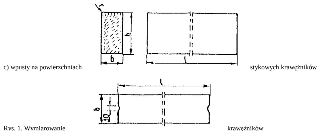
Rys. 1. Wymiarowanie
