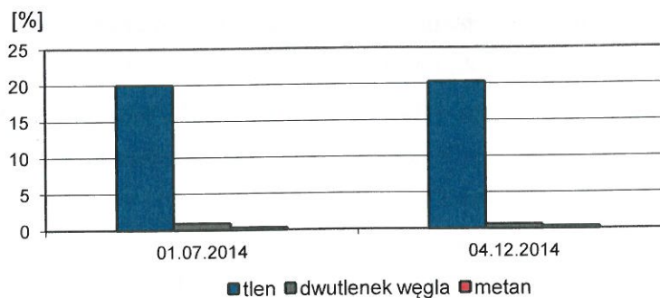
Ryc. 10. Zmienność procentowej zawartości O 2 , CO 2 i CH 4 w studziencie odgazowującej S1
