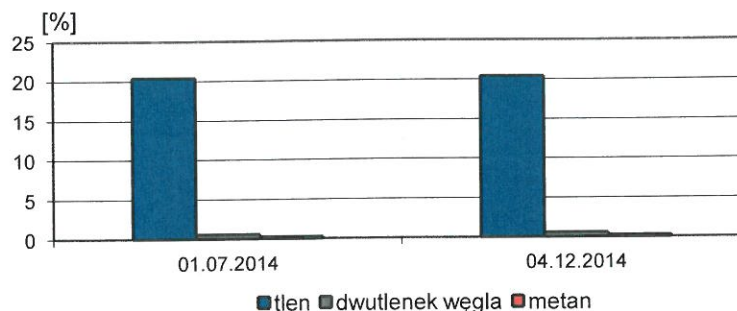
Ryc. 11 Zmienność procentowej zawartości O 2 , CO 2 i CH 4 w studziencie odgazowującej S2
