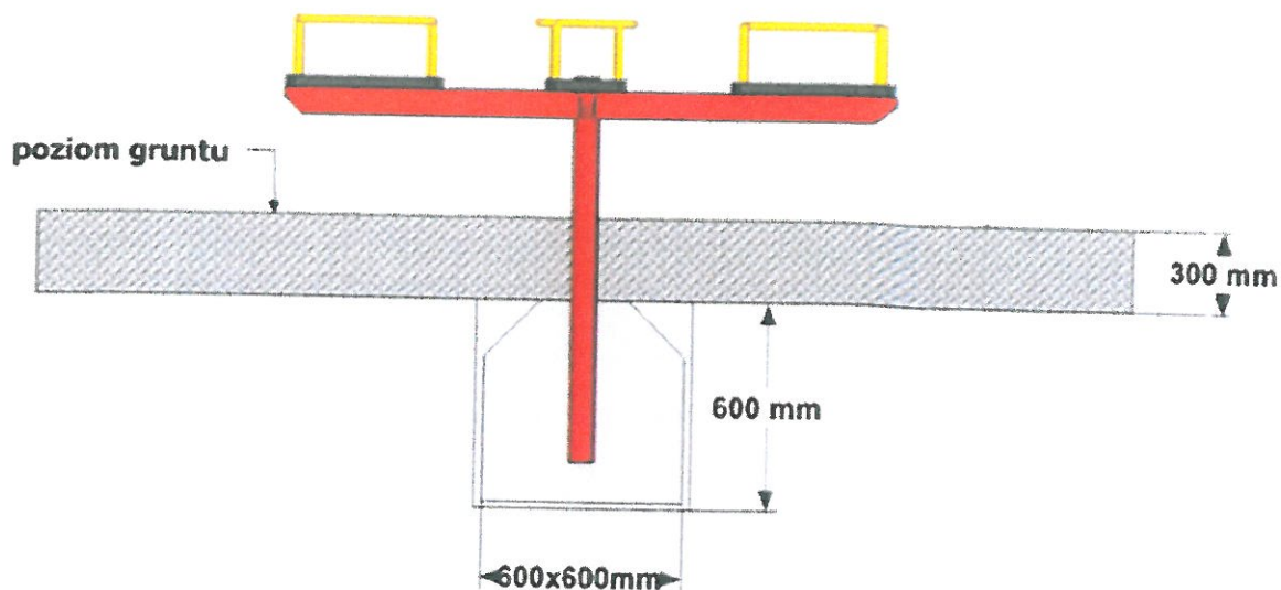
Rys. 4 Sposób montażu
