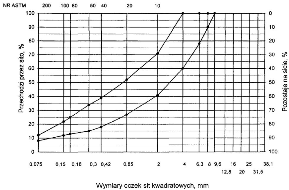
Wymiary oczek sit kwadratowych, mm Rys. 3. Krzywe graniczne uziarnienia mieszanki mineralnej BA od 0 do 8mm, od 0 do 6,3 mm do warstwy ścieralnej nawierzchni drogi o obciążeniu ruchem nawierzchni drogi o obciążeniu ruchem KR1 lub KR2
