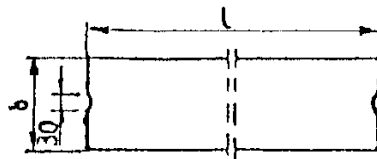
Rys. 1. Wymiarowanie krawężników
