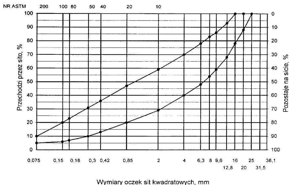
Rys. 1. Krzywe graniczne uziarnienia mieszanek mineralnych BA od 0 do 20 mm do warstwy ścieralnej nawierzchni drogi o obciążeniu ruchem dla KR1 lub KR2
