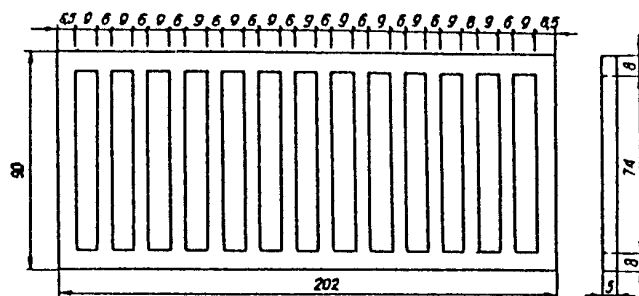
Deska ażurowa prosta 202 x 60 x 5 cm
