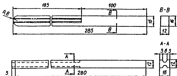
Słup dla ogrodzeń o wysokości 1,50 m
