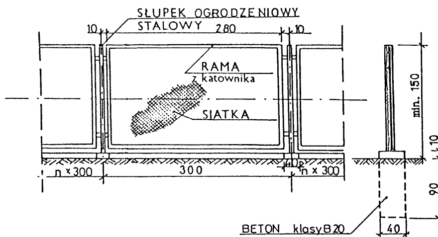
11.1.5. Brama i furtka w ogrodzeniu drogowym (wg KPED [44])
