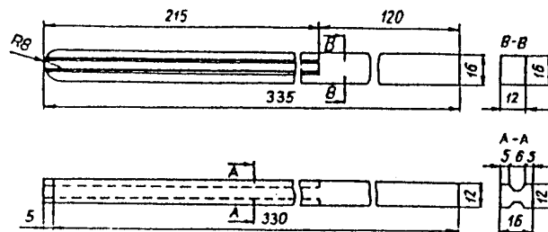
Słup dla ogrodzeń o wysokości 1,80 m
