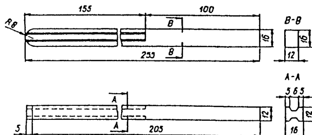
Słup dla ogrodzeń o wysokości zmiennej, szczegół przekroju poprzecznego słupa
