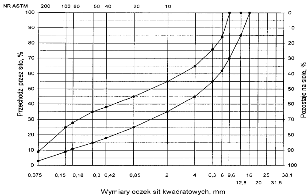
Rys. 10. Krzywe graniczne uziarnienia mieszanki mineralnej BA od 0 do 12,8 mm do warstwy wiążącej, wyrównawczej i wzmacniającej nawierzchni drogi o obciążeniu ruchem KR1
