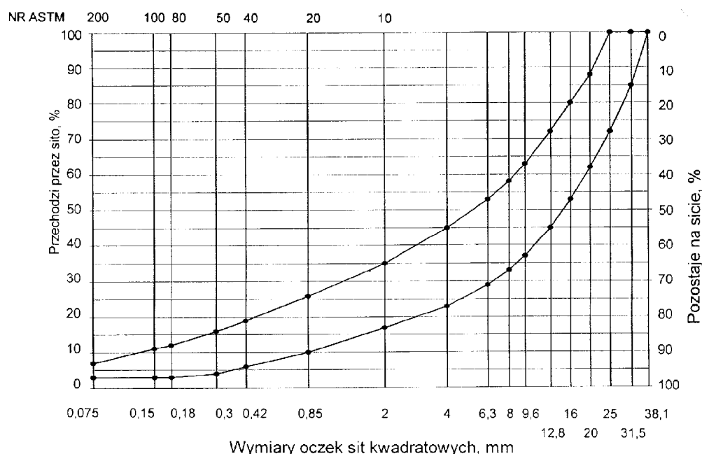
Rys.1. Krzywe graniczne uziarnienia mieszanki mineralnej BA od 0 do 31,5 mm do podbudowy nawierzchni drogi o obciążeniu ruchem KR 1
