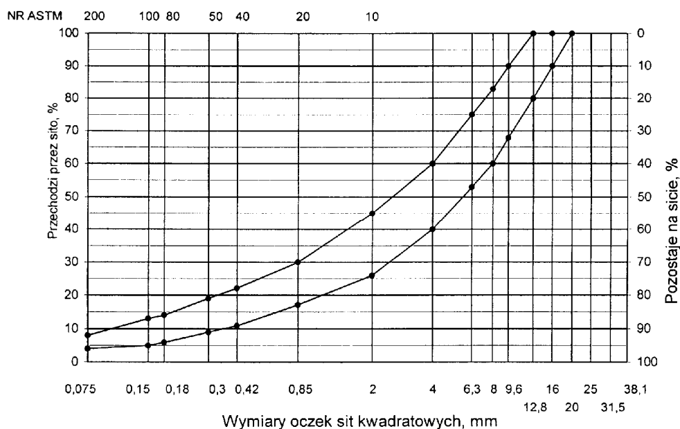
Rys. 3. Krzywe graniczne uziarnienia mieszanki mineralnej BA od 0 do 20 mm do podbudowy nawierzchni drogi o obciążeniu ruchem KR 1
