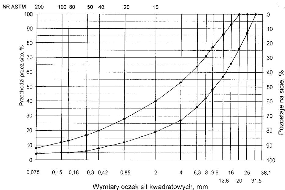
Rys. 2. Krzywe graniczne uziarnienia mieszanki mineralnej BA od 0 do 25mm do podbudowy nawierzchni drogi o obciążeniu ruchem KR 1
