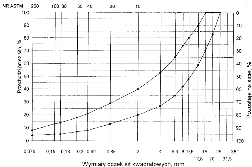
Rys. 3. Krzywe graniczne uziarnienia mieszanki mineralnej BA od 0 do 20 mm do podbudowy nawierzchni drogi o obciążeniu ruchem KR 1
